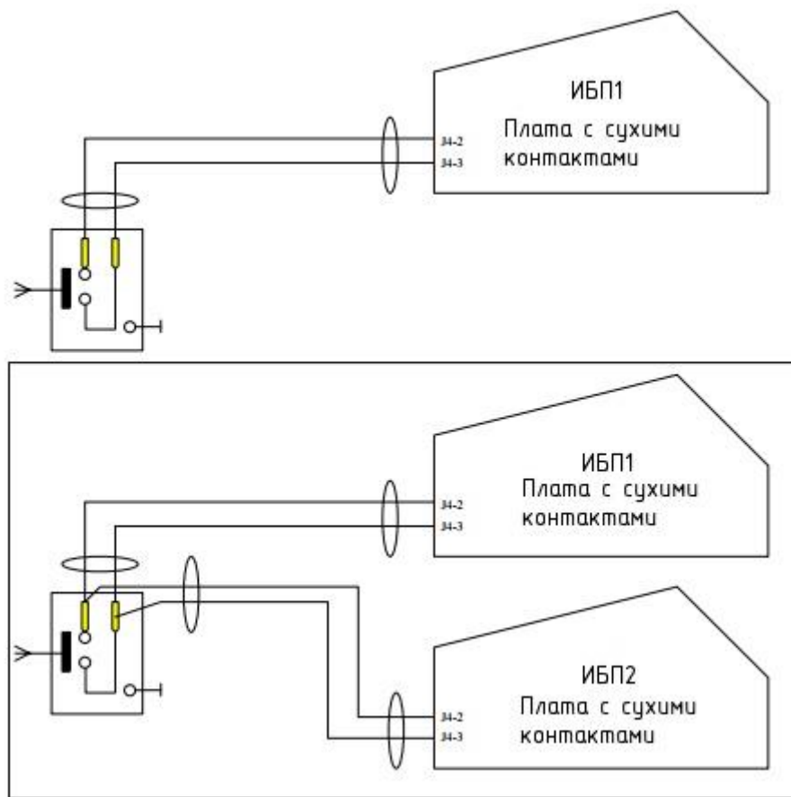
Рис. 1-21 Контур EPO
