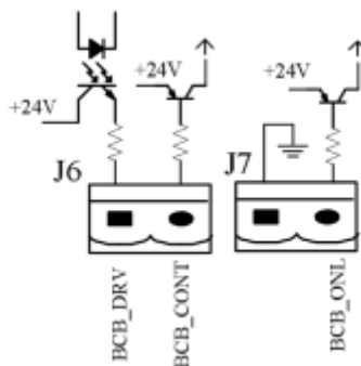
Рис. 1-15. Интерфейс ВСВ
