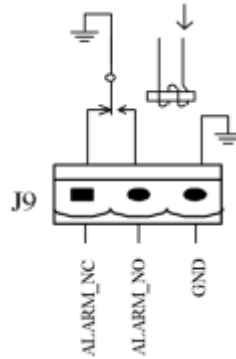
Рис. 1-17. Схема интерфейса с сухими контактами для объединенного предупреждения
