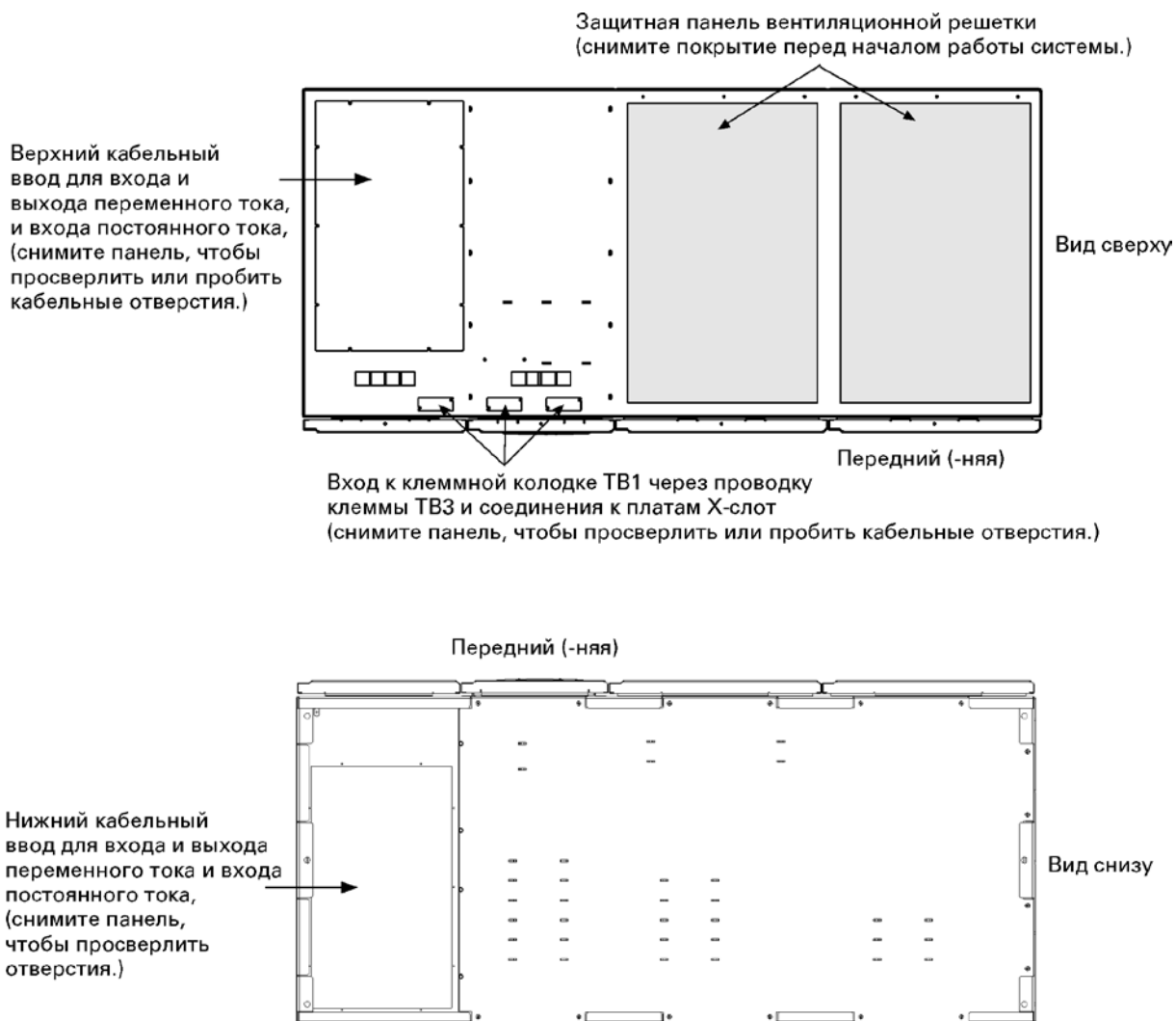
Рис. 3-3. Местоположение входов кабелей
