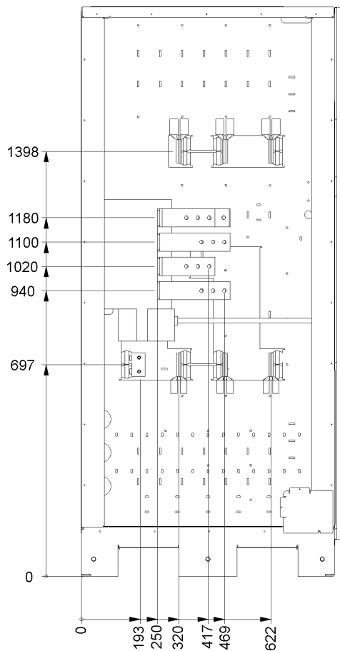
Figure 3-5b. Вид сзади (или со стороны) , Местоположение силовых клемм ИБП
