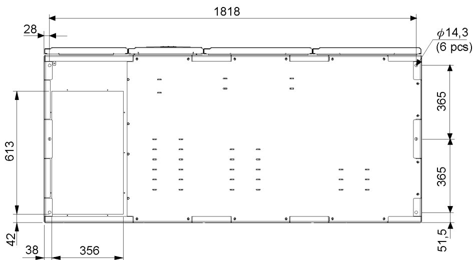
Рис. 2-4. Размеры ИБП (вид снизу)
