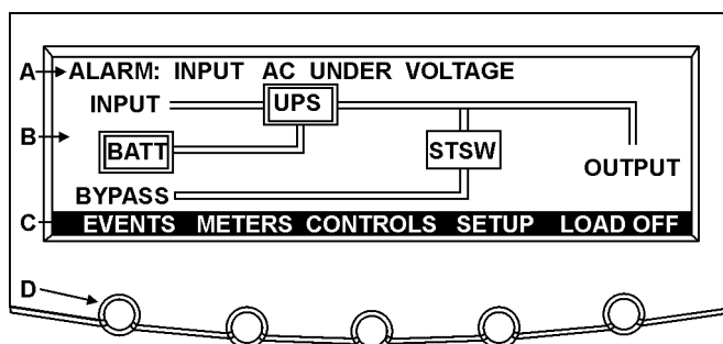
Рис. 5-3. Зоны ЖК-дисплея.
