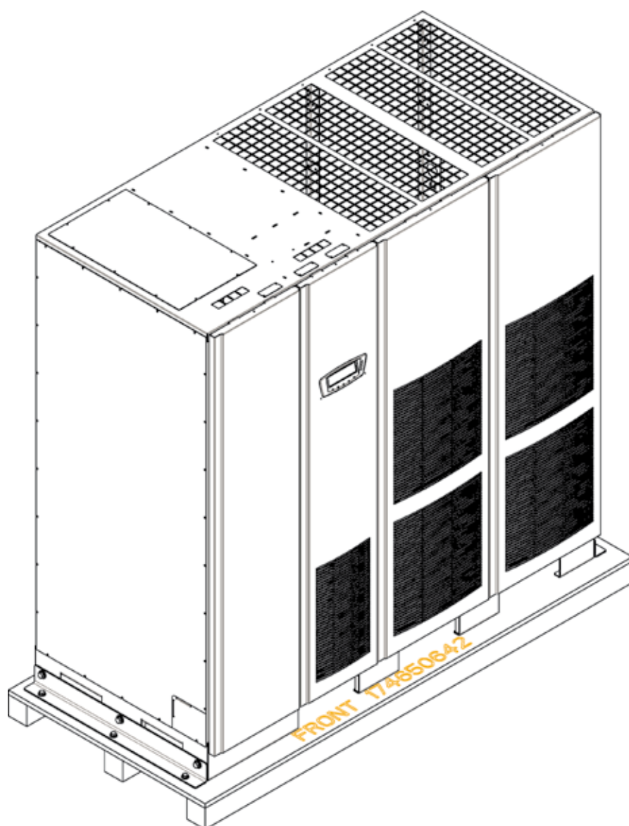
Рис. 2-8. Шкаф ИБП Powerware 9395 (2x275 кВА) при транспортировке на поддоне
