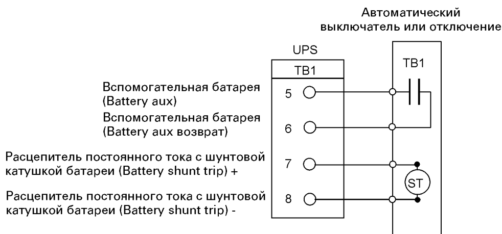
Рис. 3-10. Подключение сигнальных батарейных кабелей устройств к батарее
