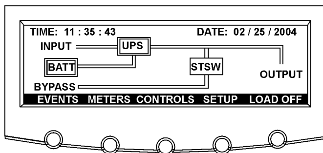
Рис. 5-4. Основное меню и мнемосхема (нормальный режим).
