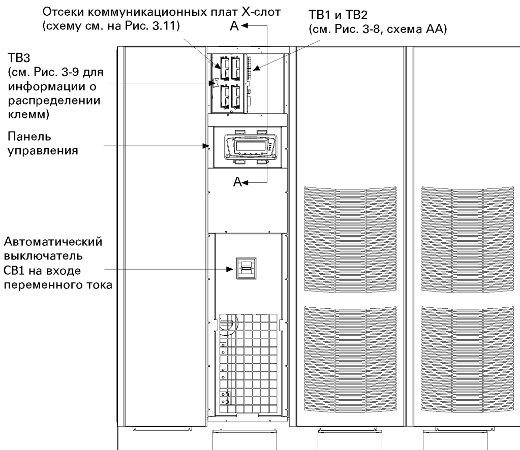
Рис. 3-7. Расположение клемм для подключения внешних устройств
