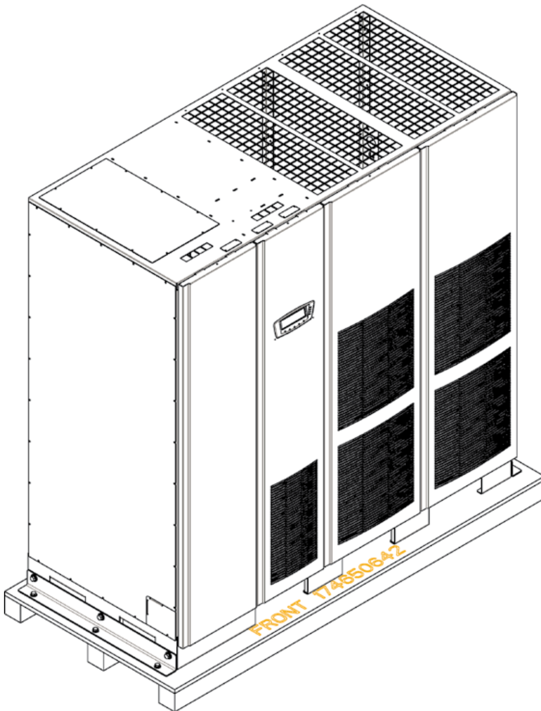
Рис. 1-1. Шкаф ИБП Powerware 9395-550 (2x275 кВА)
