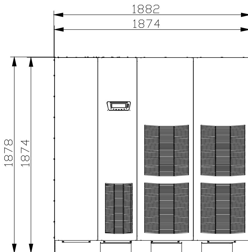
Рис. 2-1. Размеры ИБП (вид спереди)
