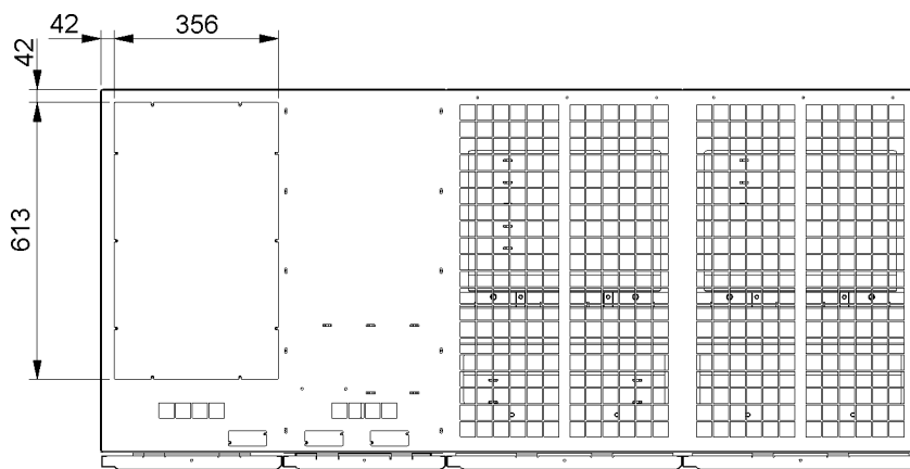
Рис. 2-3. Размеры ИБП (вид сверху)
