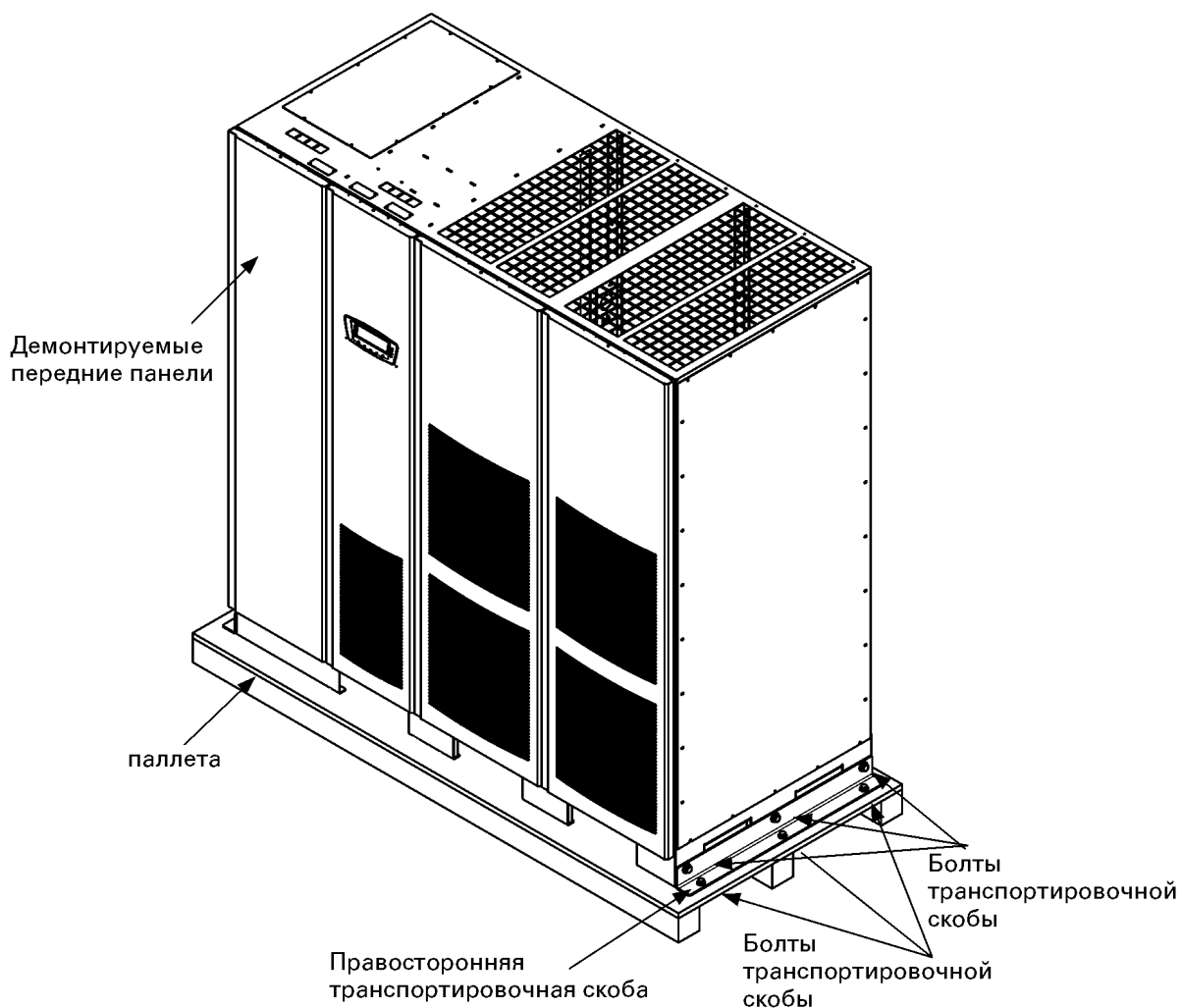
Рис. 3-2. Демонтаж правой транспортировочной скобы
