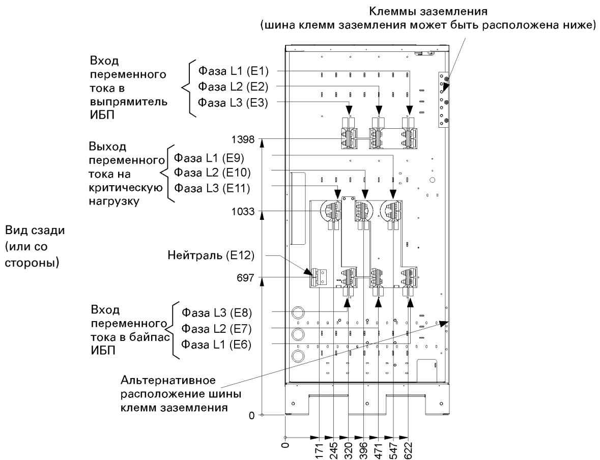
Рис. 3-4б. Местоположение силовых клемм ИБП
