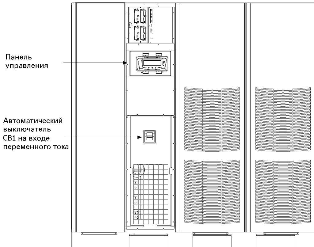
Рис. 5-1. Кнопки управления и индикаторы ИБП Powerware 9395 450-550 кВА
