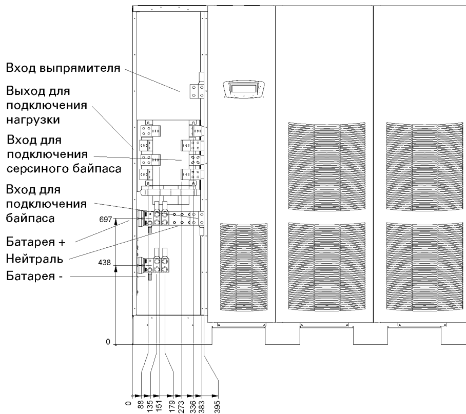
Figure 3-5a. Вид спереди
