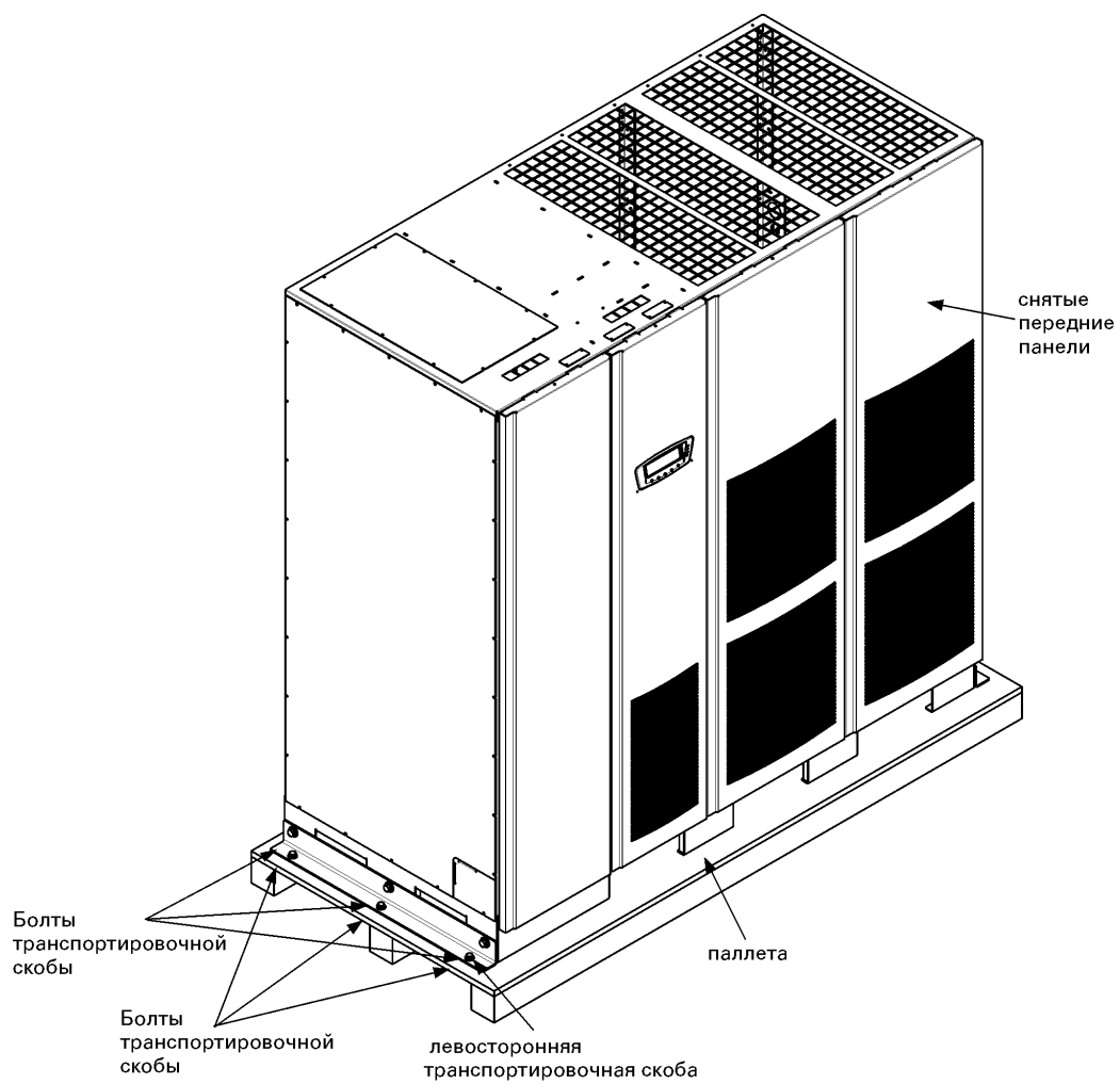
Рис. 3-1. Демонтаж левой транспортировочной скобы
