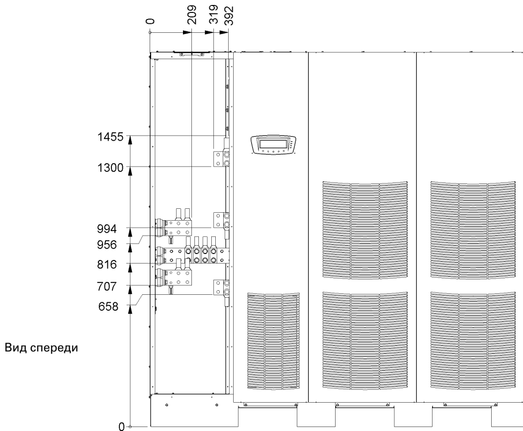
Рис. 3-4а. Местоположение силовых клемм ИБП
