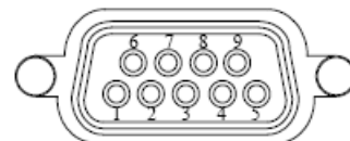
Рис. 8-1 Назначение контактов
